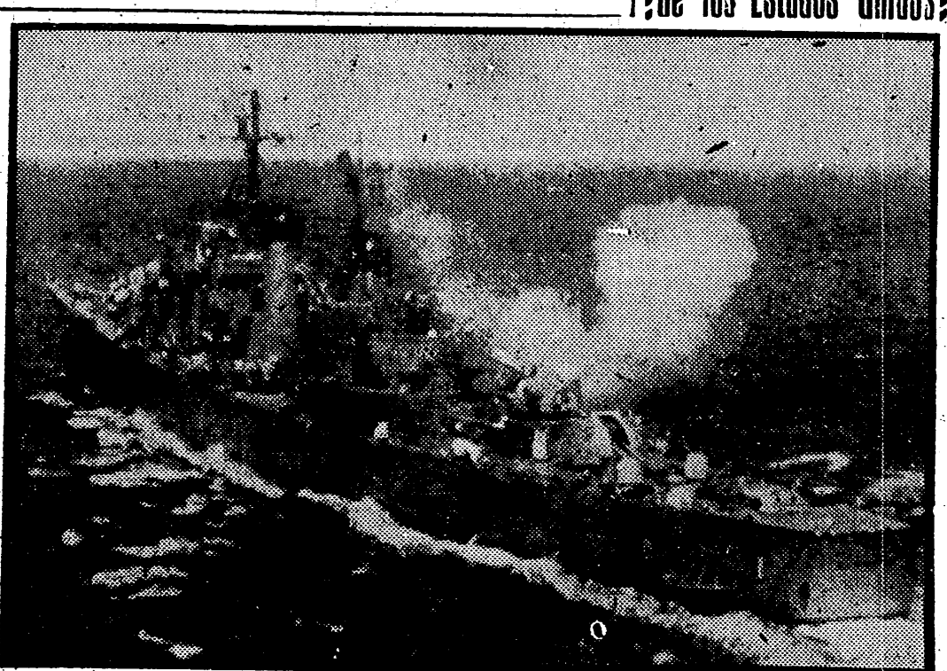
ESTADOS UNIDOS. — Un buque de la Marina norteamericana en el momento de lanzar un proyectil dirigido anti-submarino "Asroc", durante unas pruebas realizadas con gran éxito con el nuevo torpedo.
