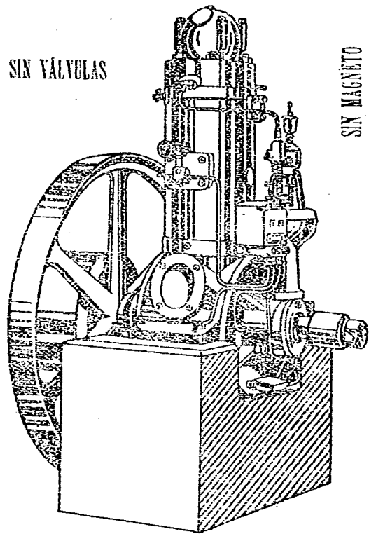
SEMI-DIESEL a 2 tiempos
